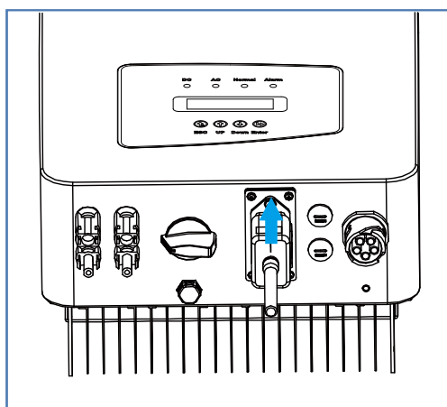
Rys. 5.13 Schemat instalacyjny rejestratora danych
