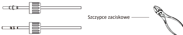
Rys. 5.4 Zaciśnij pin kontaktowe do przewodu
