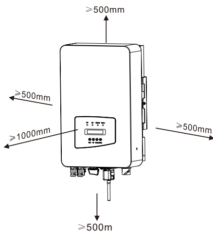
Rys. 4.3 Przerwa Instalacyjna
