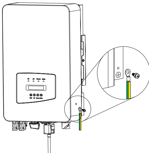
Rys. 5.11 Instalacja obudowanego przewodu uziemiającego
