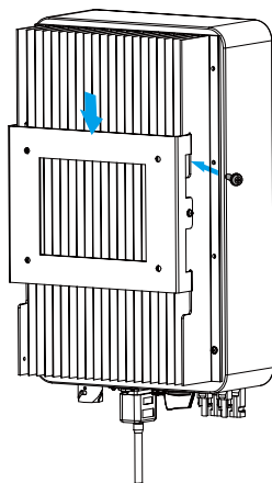
Rys. 4.6 Instalacja Inwertera
